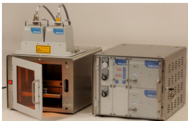
Die Belichtungskammer und die Steuerung kann bis zu 2m auseinander aufgestellt werden
